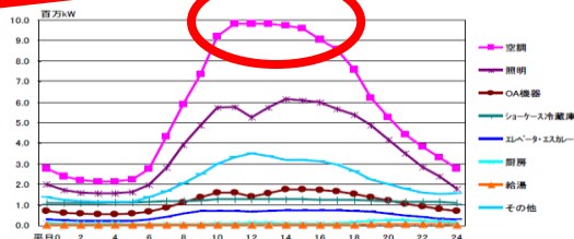
【時間帯別電力需要(機器別)】
